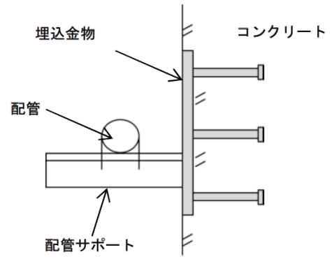
配管サポート固定イメージ
