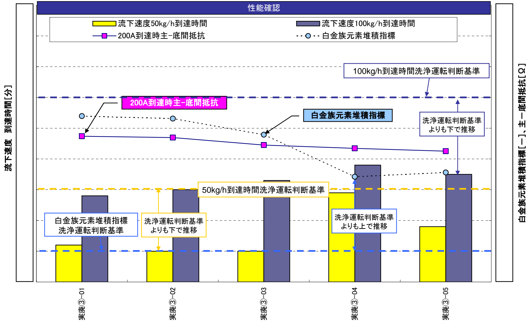
図一Ⅲ. 2. 2. 9 A系列性能確認での流下性指標等の推移
