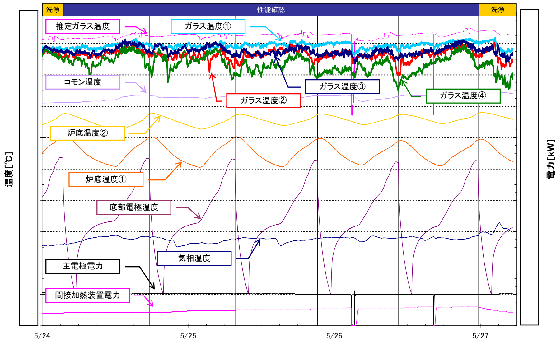
図一Ⅲ. 2. 2. 7 A系列性能確認でのガラス温度等の推移
