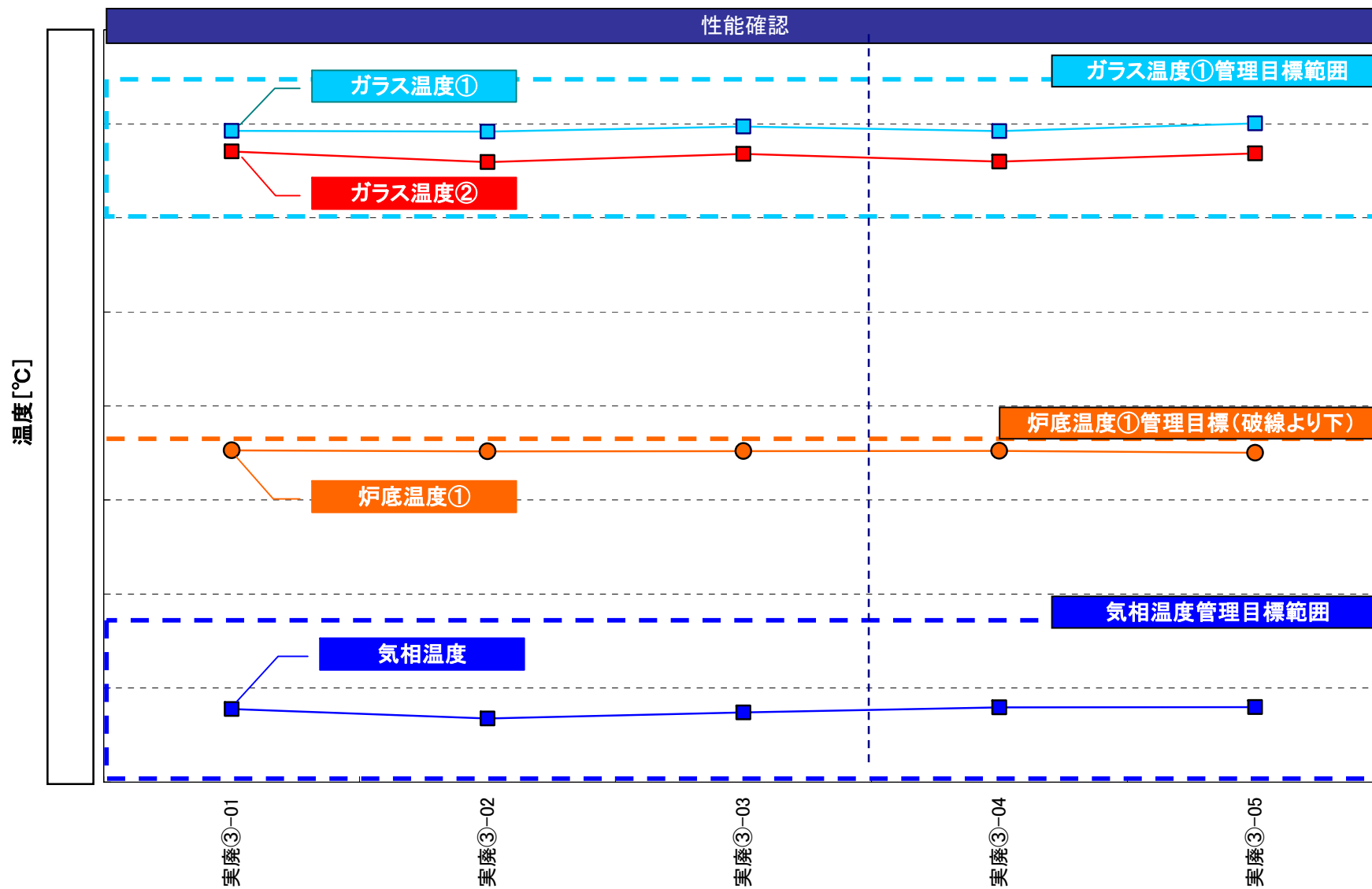
図-Ⅲ. 2. 2. 8 A系列性能確認でのガラス温度等の推移 (バッチ平均)
