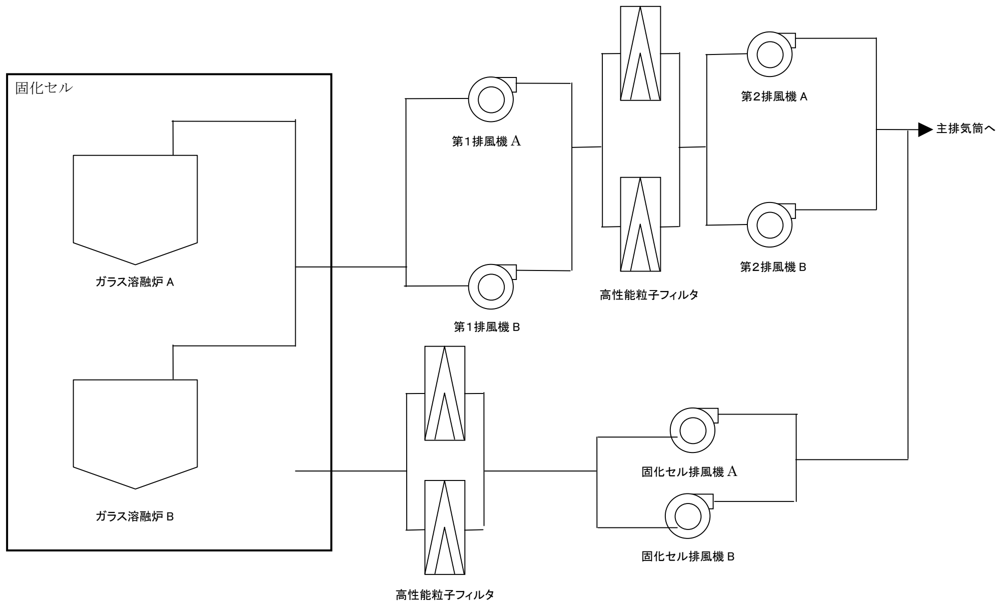
高レベル廃液ガラス固化建屋 高レベル廃液ガラス固化廃ガス処理設備の概略図
