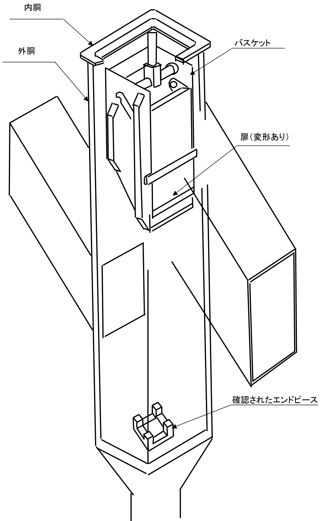
エンドピース酸洗浄槽の状況図
