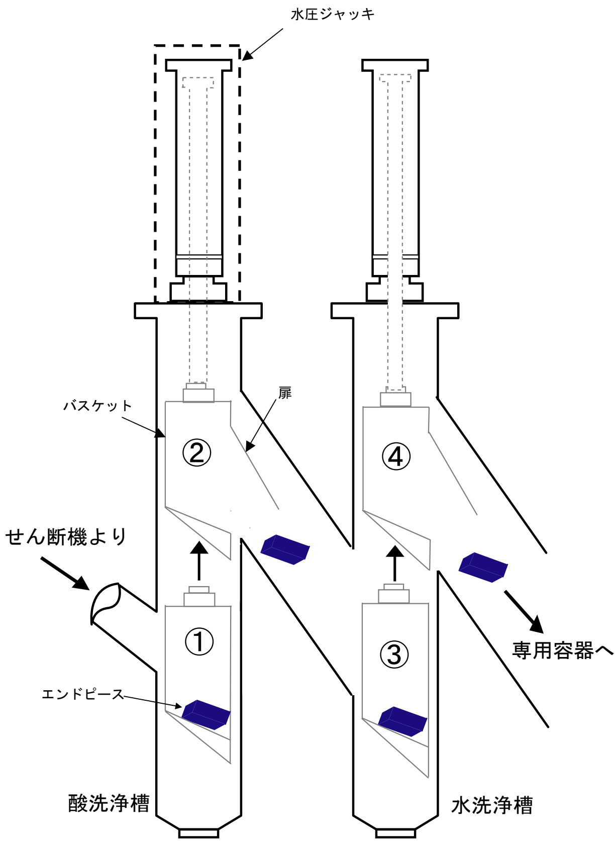
エンドピース酸洗浄槽、水洗浄槽でのエンドピースの流れ
