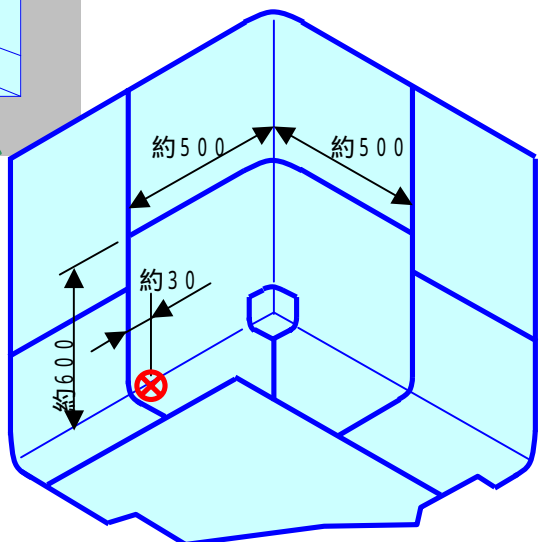
バーナブルポイズン取扱ピット 漏えい箇所
