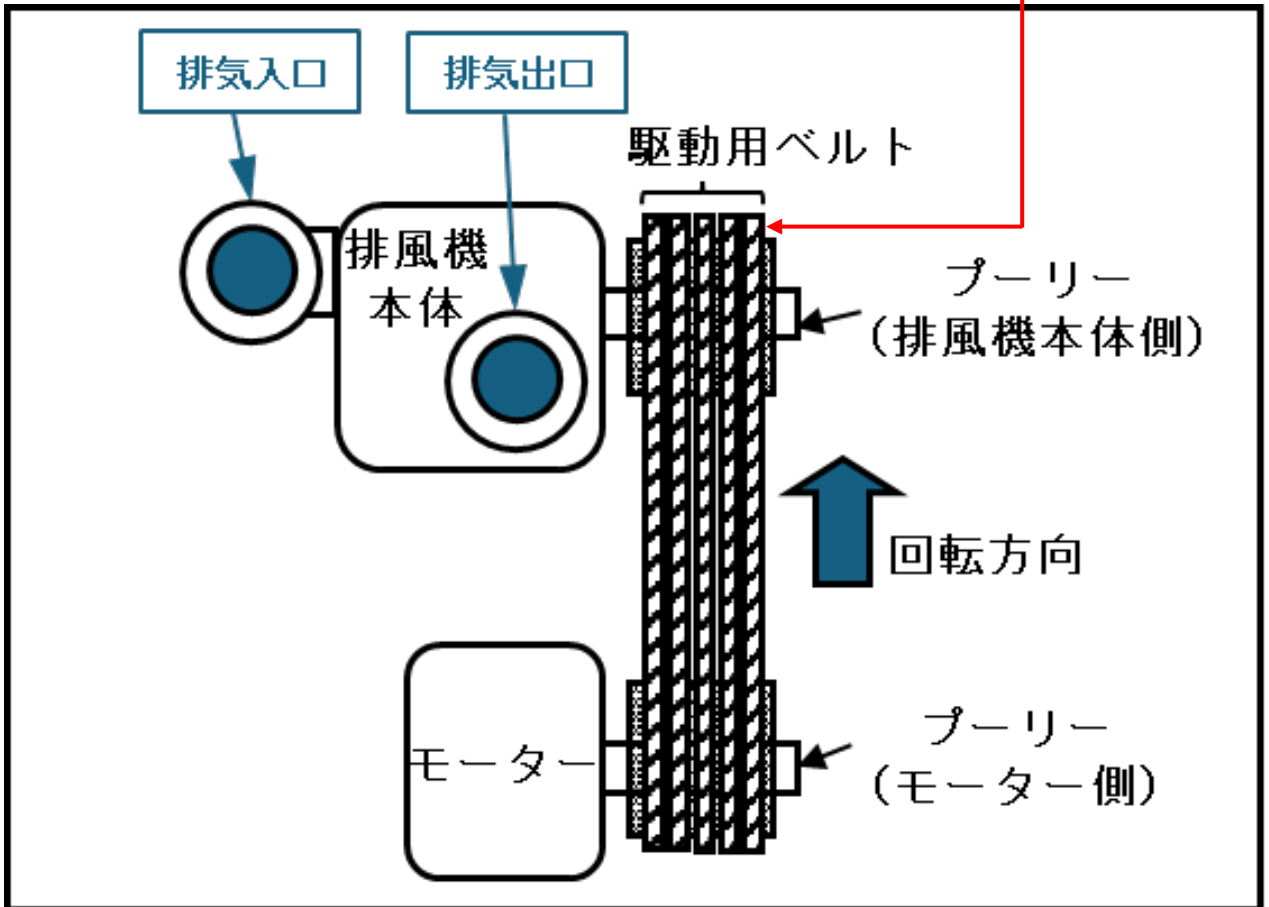
《上面図》
