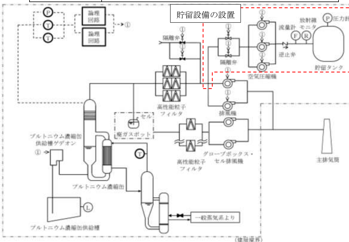
第4図 精製建屋のT B P 等の錯体の急激な分解反応に対処するための措置の系統概要図
