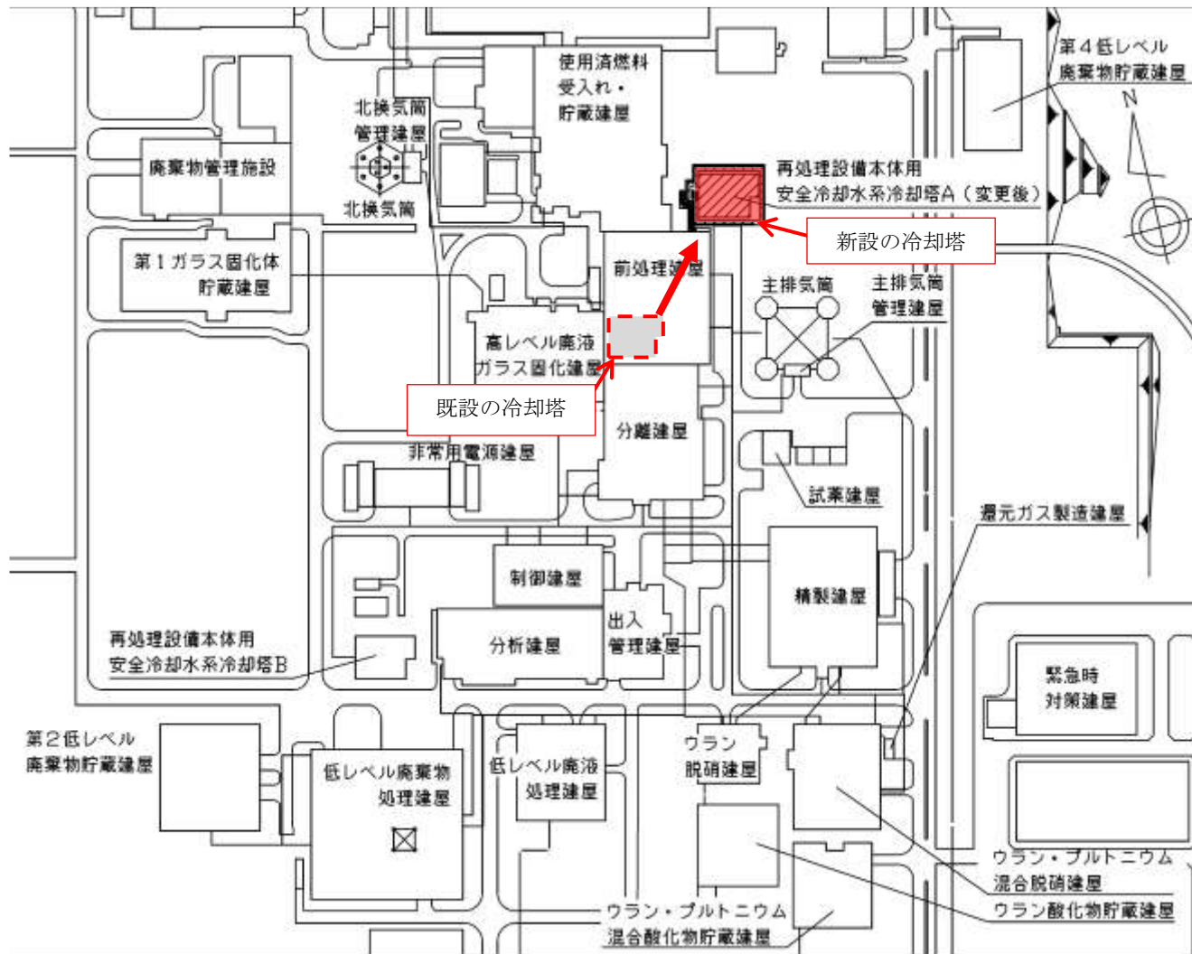
第1図 安全冷却水系冷却塔 構内配置図
