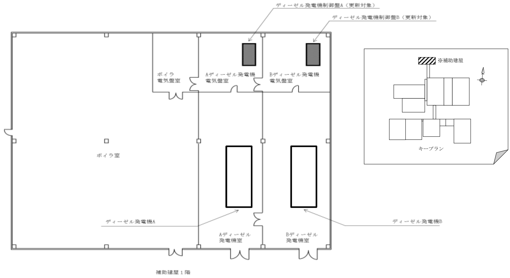
ディーゼル発電機制御盤 機器配置
