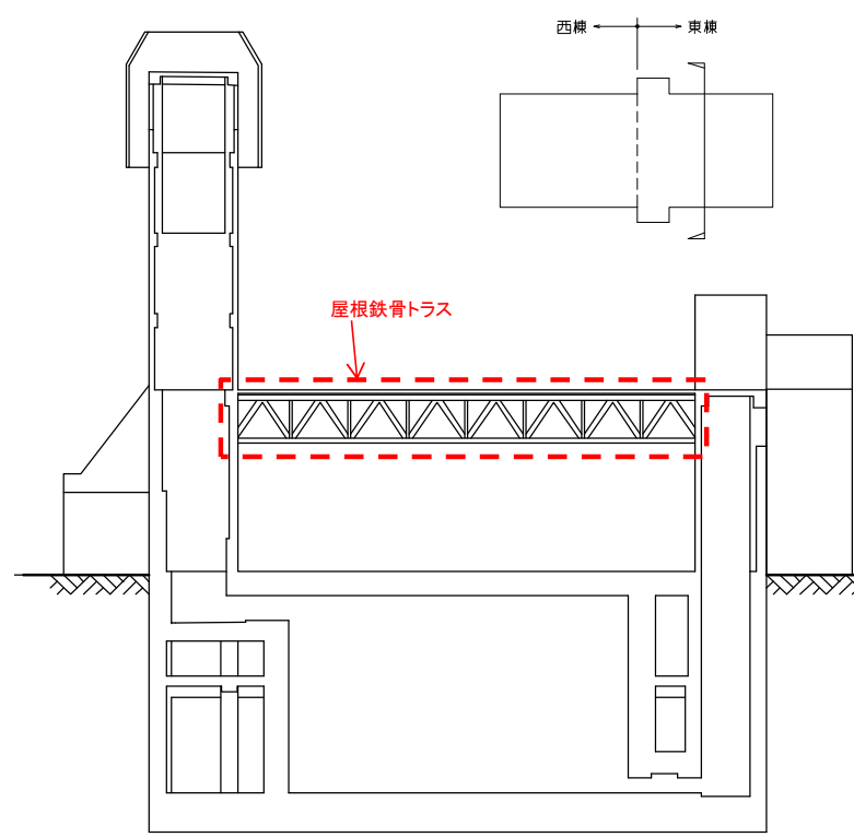
図2 第1ガラス固化体貯蔵建屋東棟 断面図
