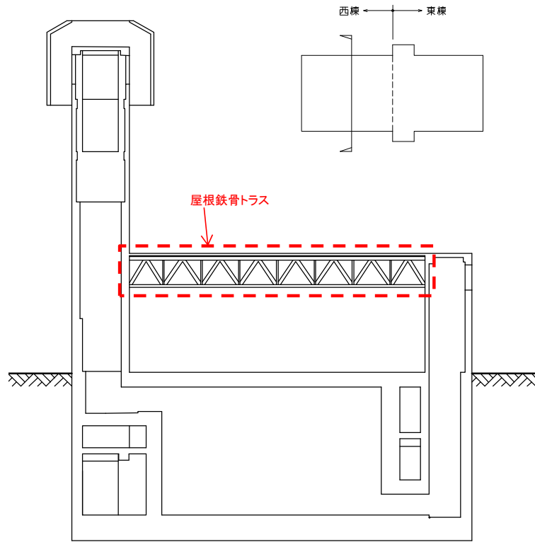
図1 第1ガラス固化体貯蔵建屋西棟 断面図
