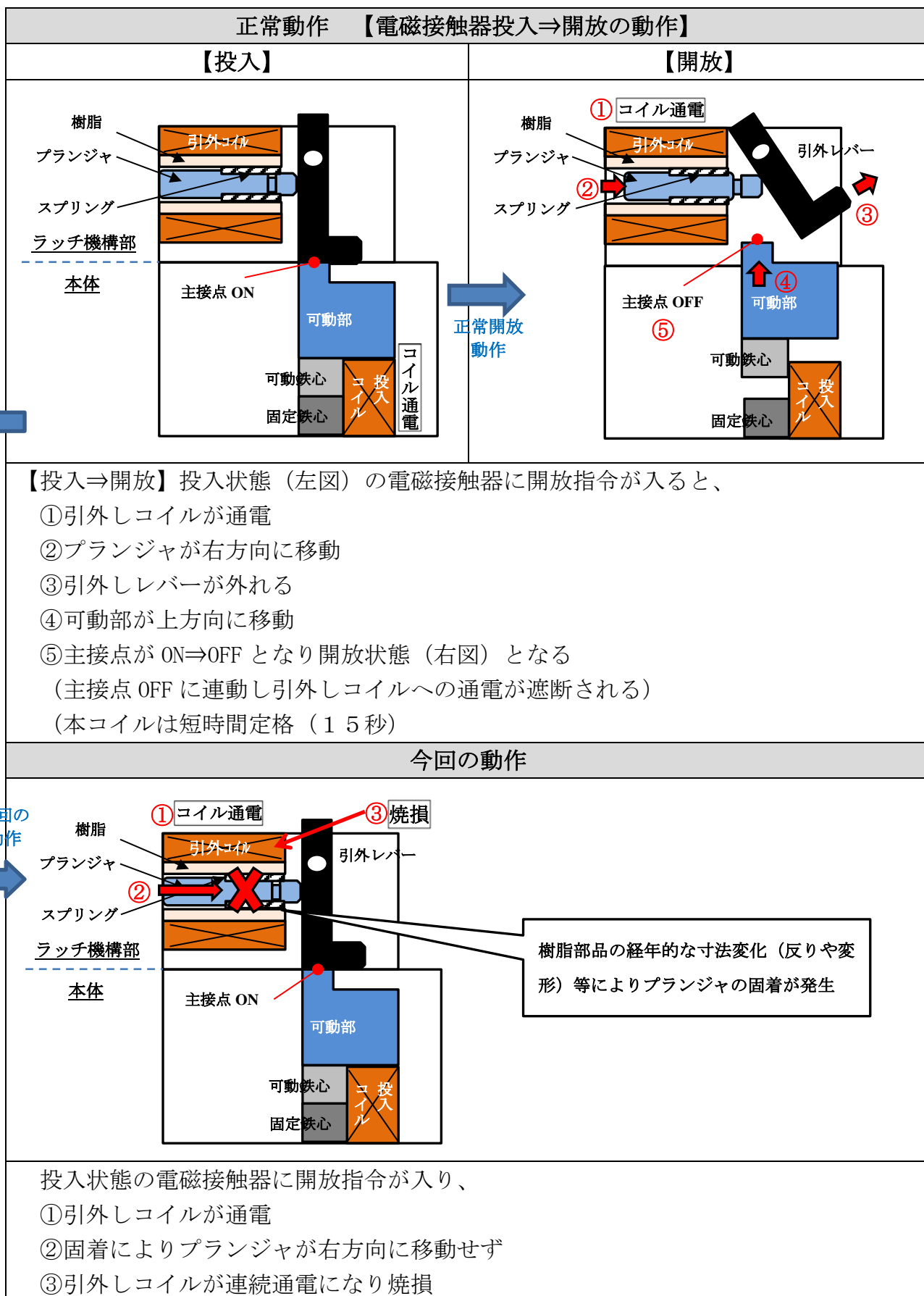
電磁接触器概要図
