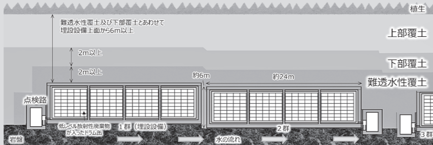
1号廃棄物埋設施設の構造
