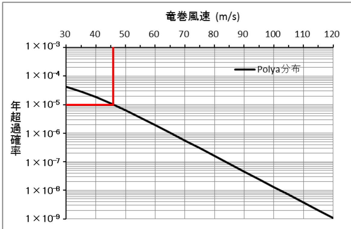
第 1.2.9-3 図 竜巻最大風速のハザード曲線(竜巻検討地域)
