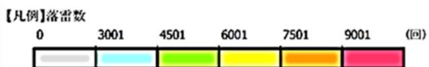
第 1.2.11－2 図 青森県の落雷密度の調査結果
