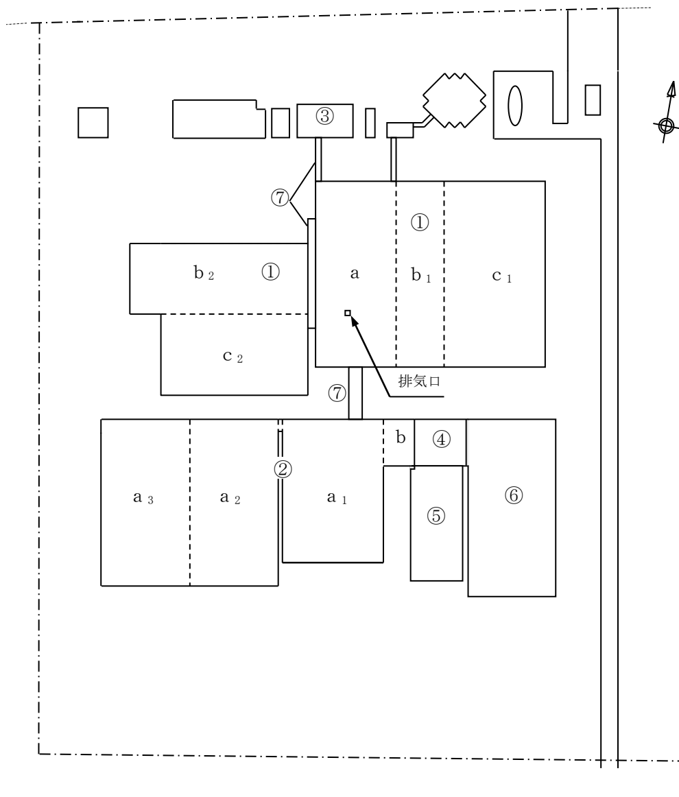
第 1.3.1-3 図 加工施設一般配置概要図
