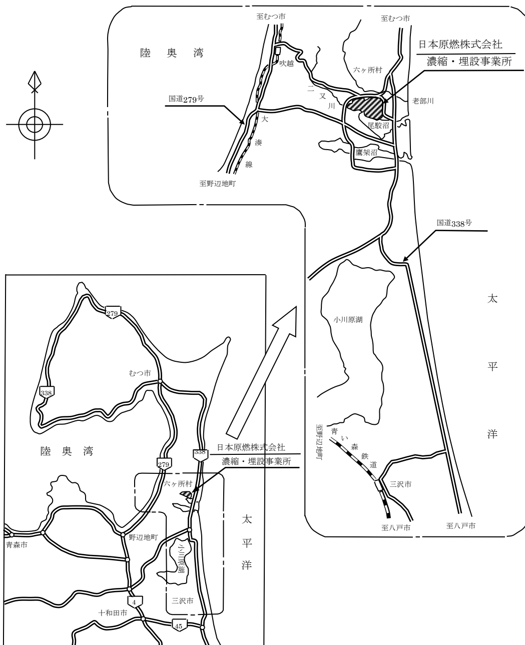
第 1.3.1-1 図 敷地付近概要図
