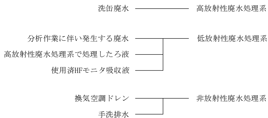
第 1.1.2－2 図 液体廃棄物の処理系統
