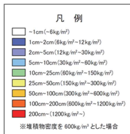
第 1.2.8-1 図 降下火砕物シミュレーションの解析結果 (風向の不確かさの考慮)
