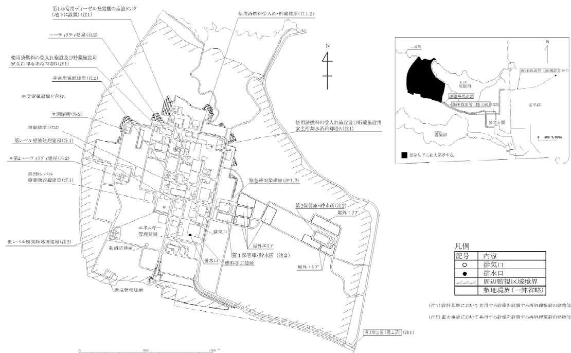
図 3-1 再処理事業所の敷地図
