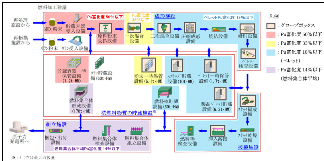
図 6-1 MOX燃料の加工工程
