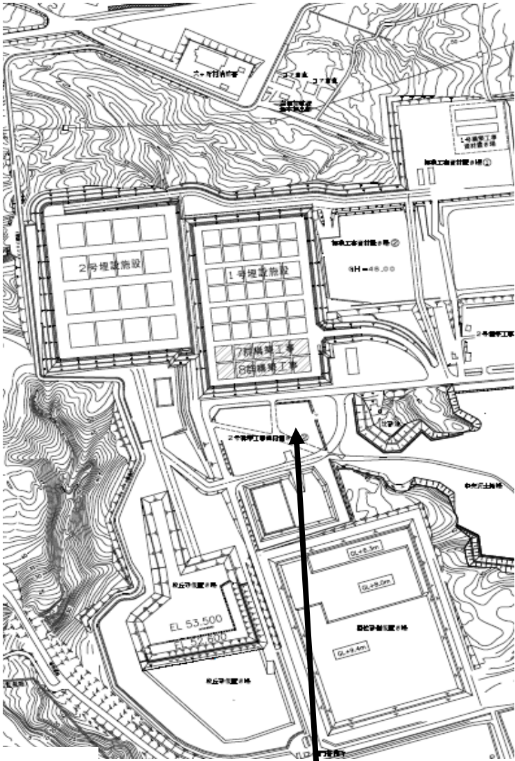
六ヶ所低レベル放射性廃棄物埋設センター構内配置図
