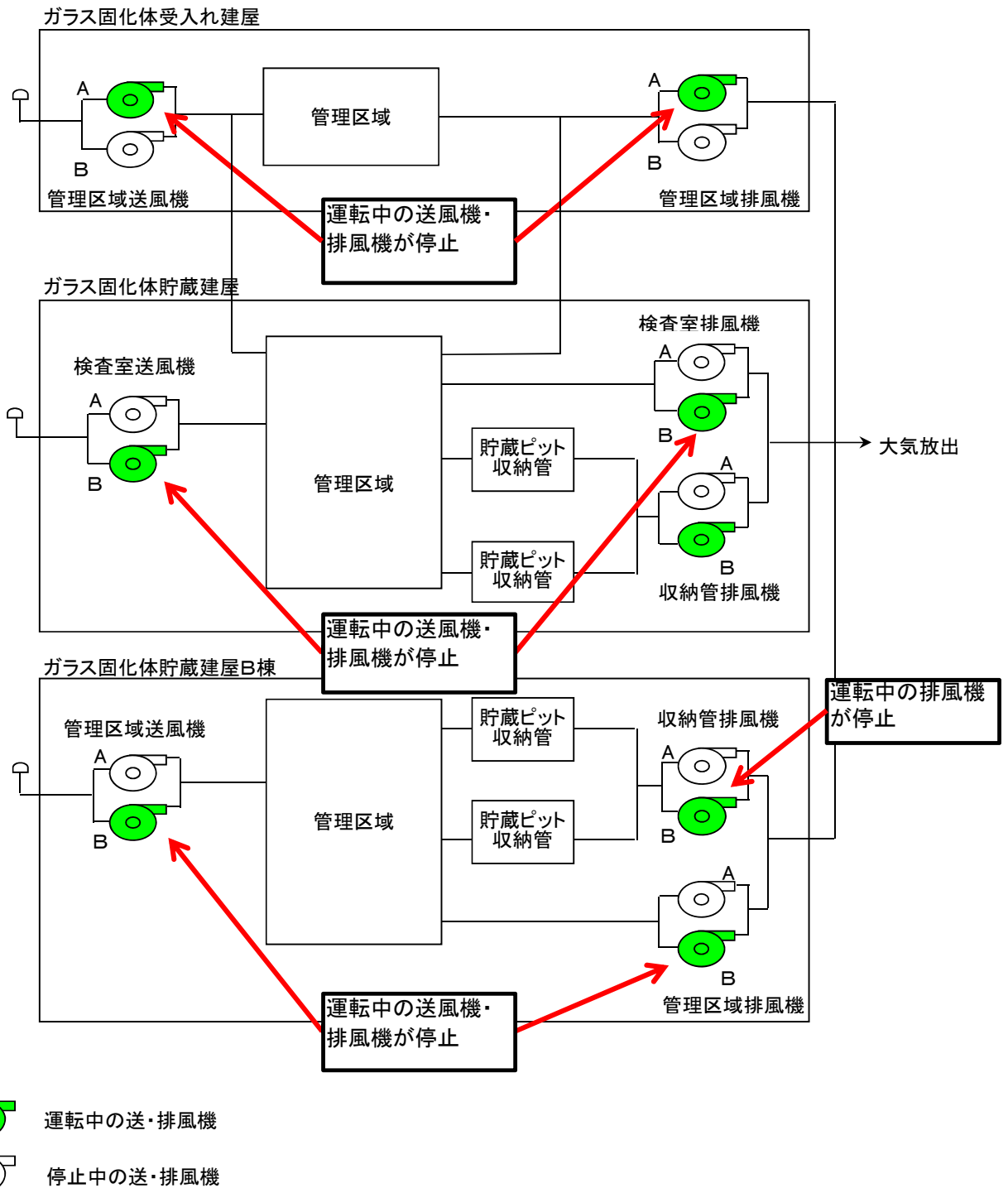
高レベル廃棄物貯蔵管理センター 換気設備概要図
