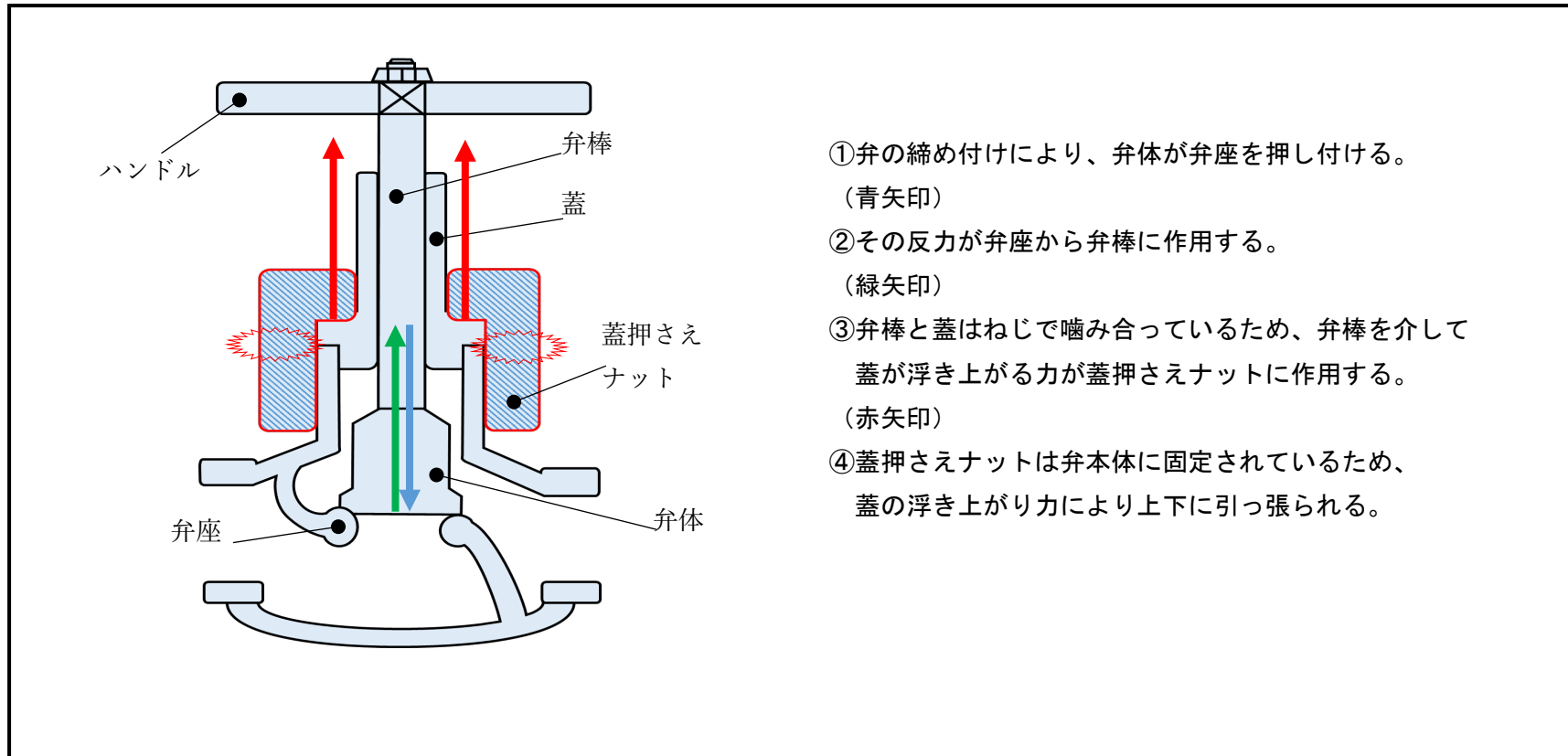
弁の締めすぎによる破損メカニズム
