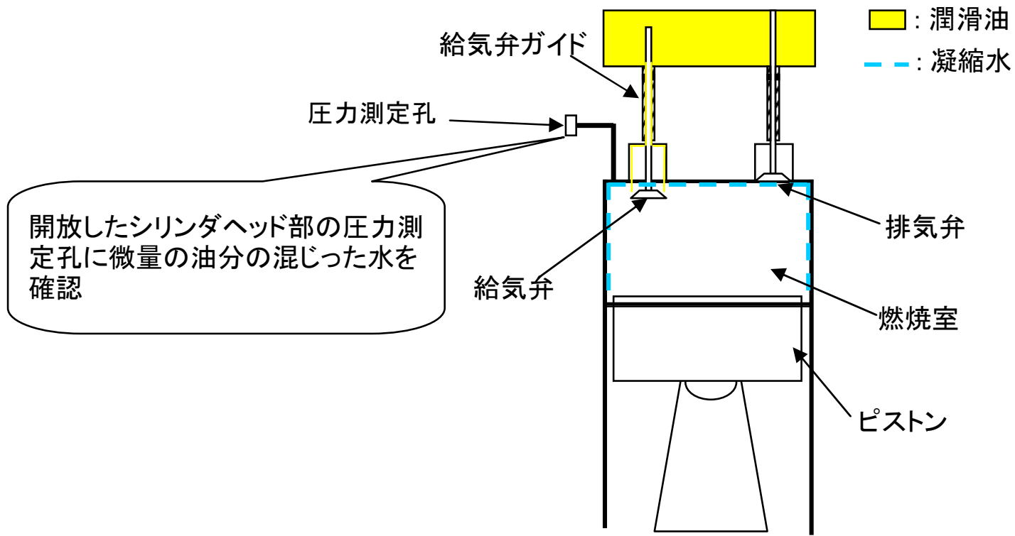
第1非常用ディーゼル発電機A号機シリンダヘッド部の概要図
