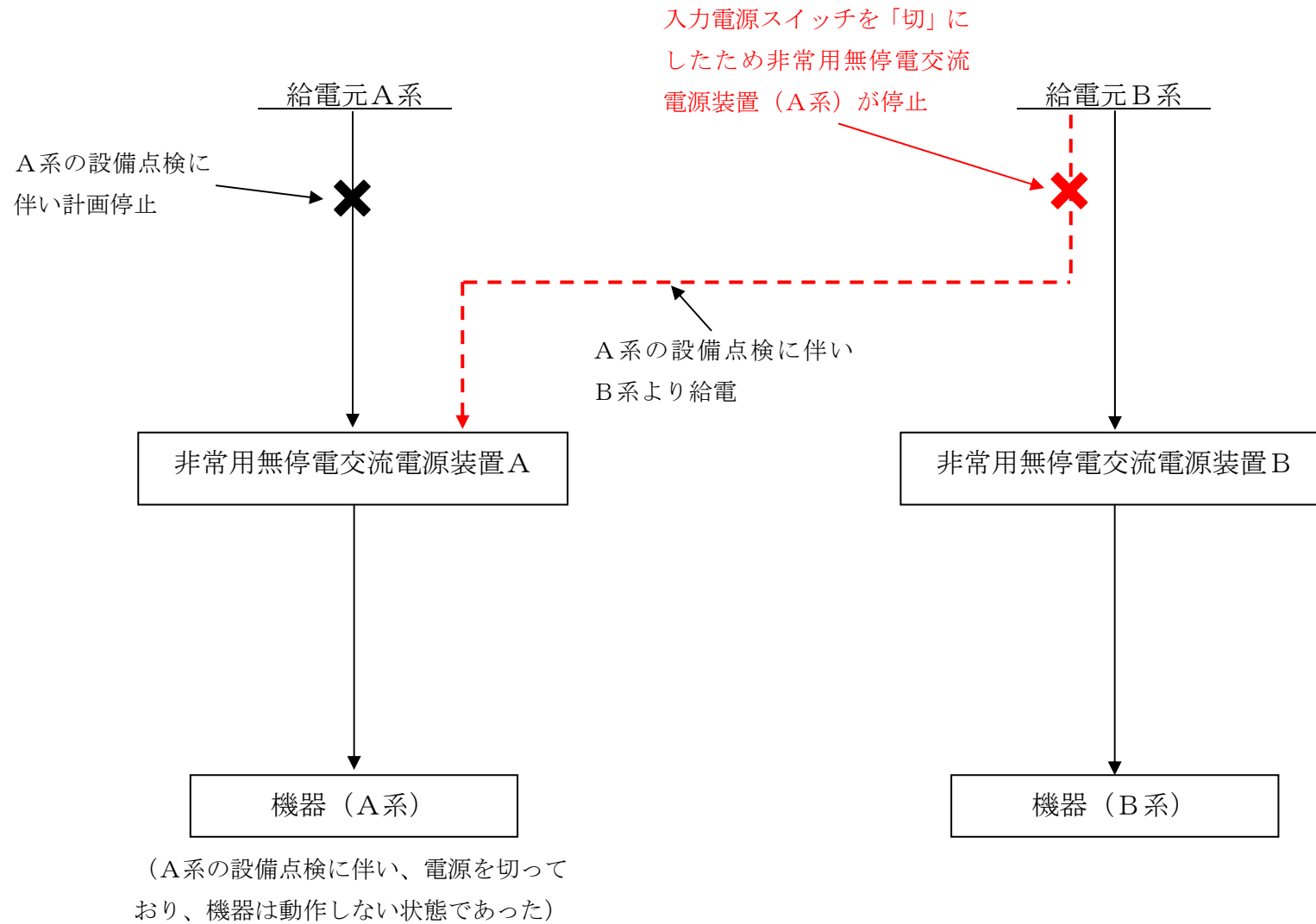
非常用無停電交流電源装置概要図
