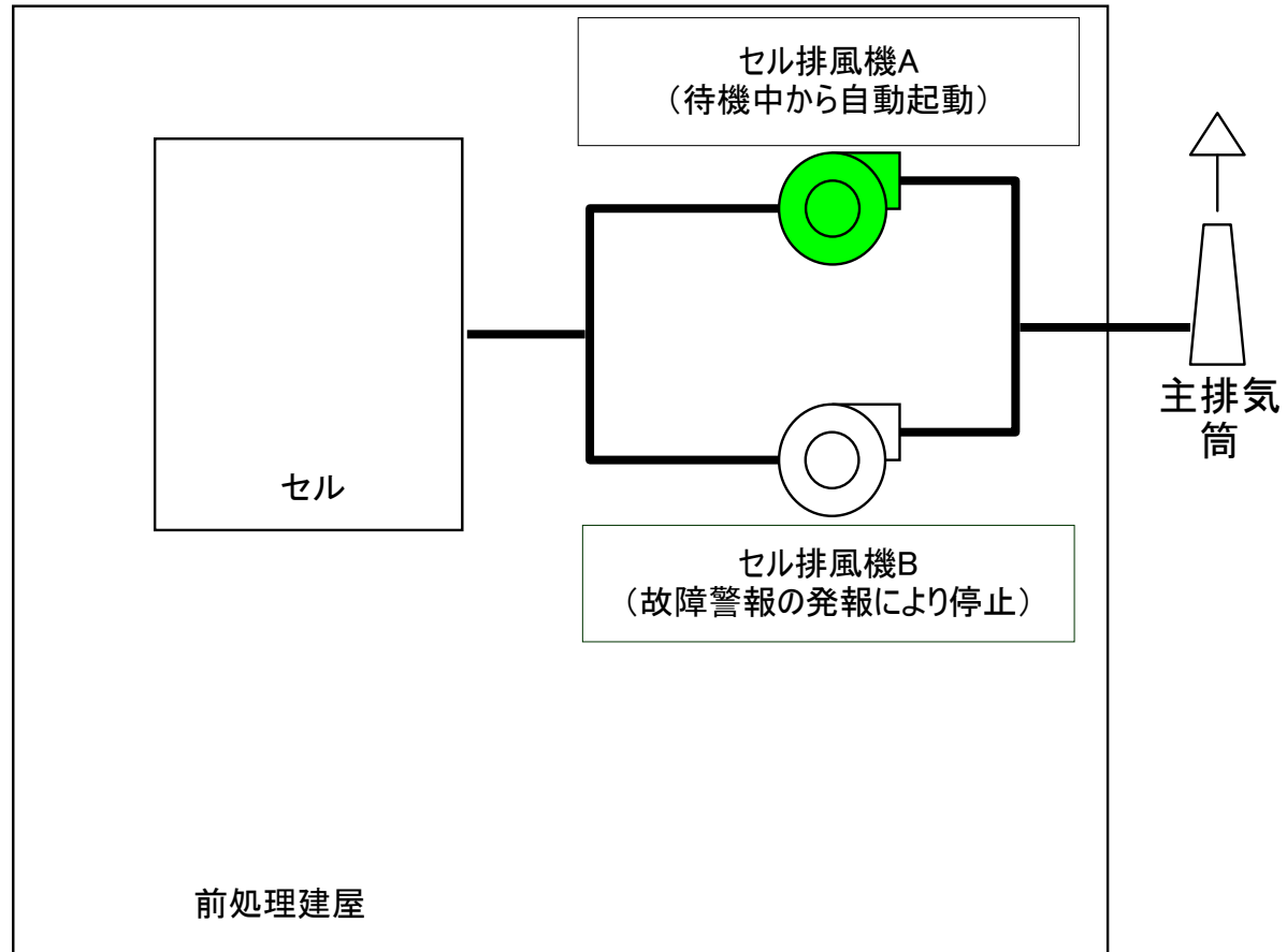
セル排風機系統概要図
