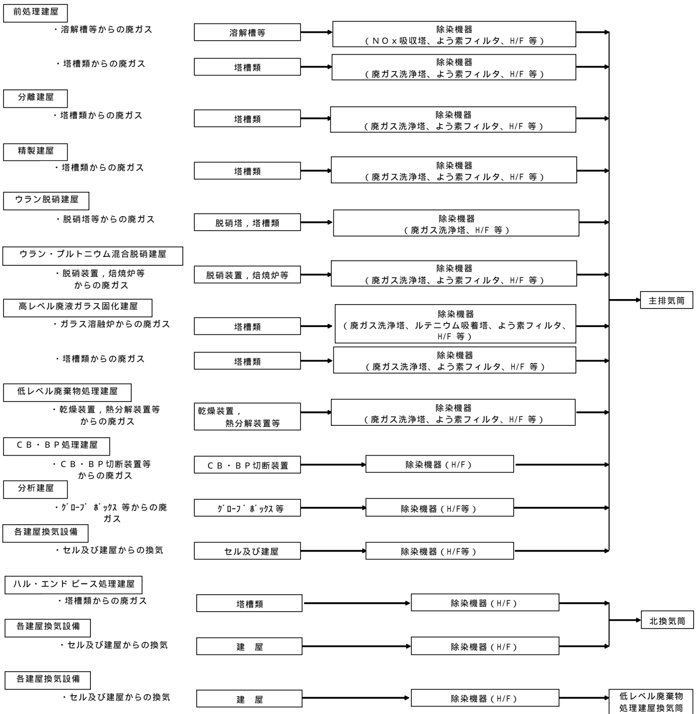
図 - 5 気体廃棄物の処理系統図 気体廃棄物の処理系統図
