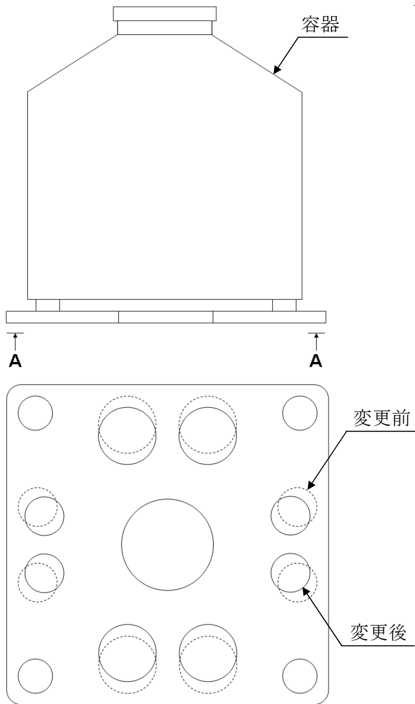
A-A 矢視
