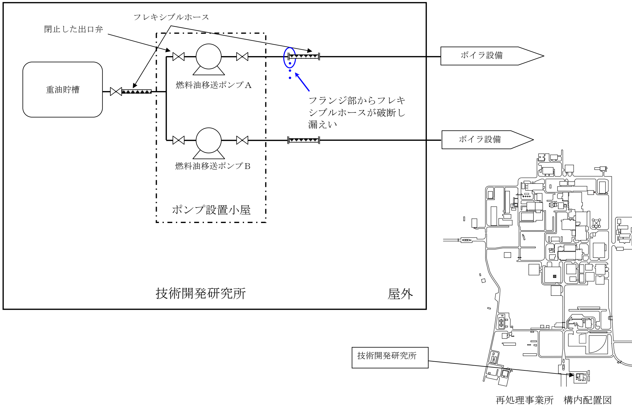
添付1 技術開発研究所屋外のボイラ用重油配管からの漏えい(概要図)
