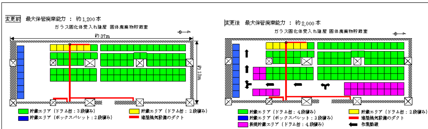
図-3 高レベル放射性廃棄物貯蔵管理センターの保管廃棄能力向上の概要
