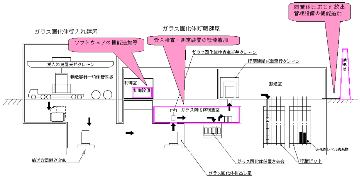
図ー２ 高レベル放射性廃棄物貯蔵管理センターの機能追加等の概要
