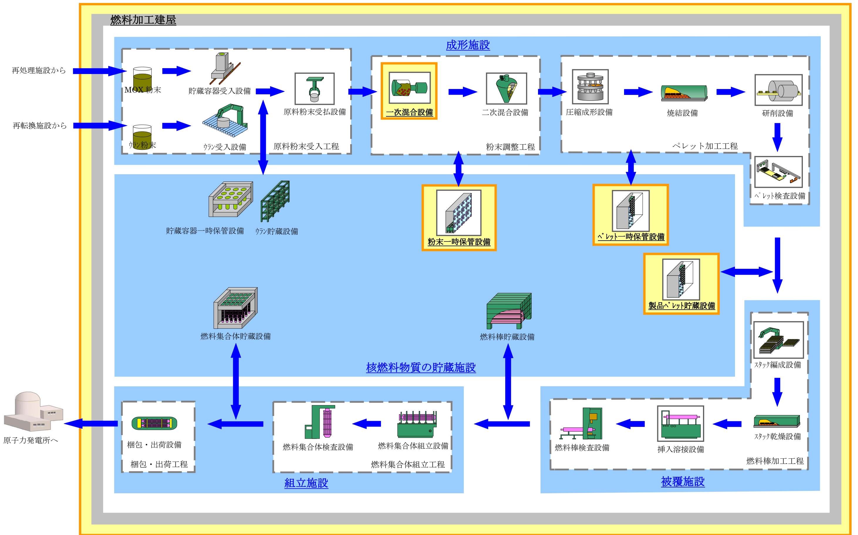
MOX燃料加工施設の概要
