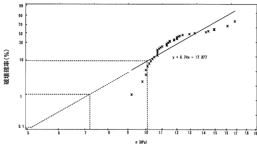
図6 内部亀裂試験データのワイブルプロット（600℃の曲げ強さ、多重モードワイブル分布）
