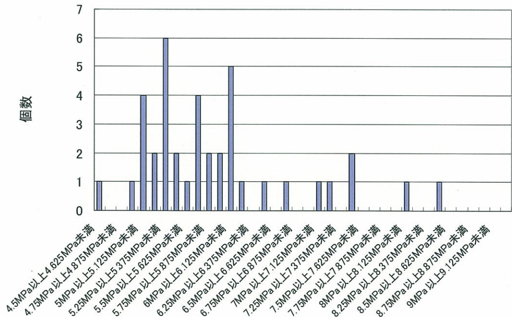
図 4 引張強度への換算
