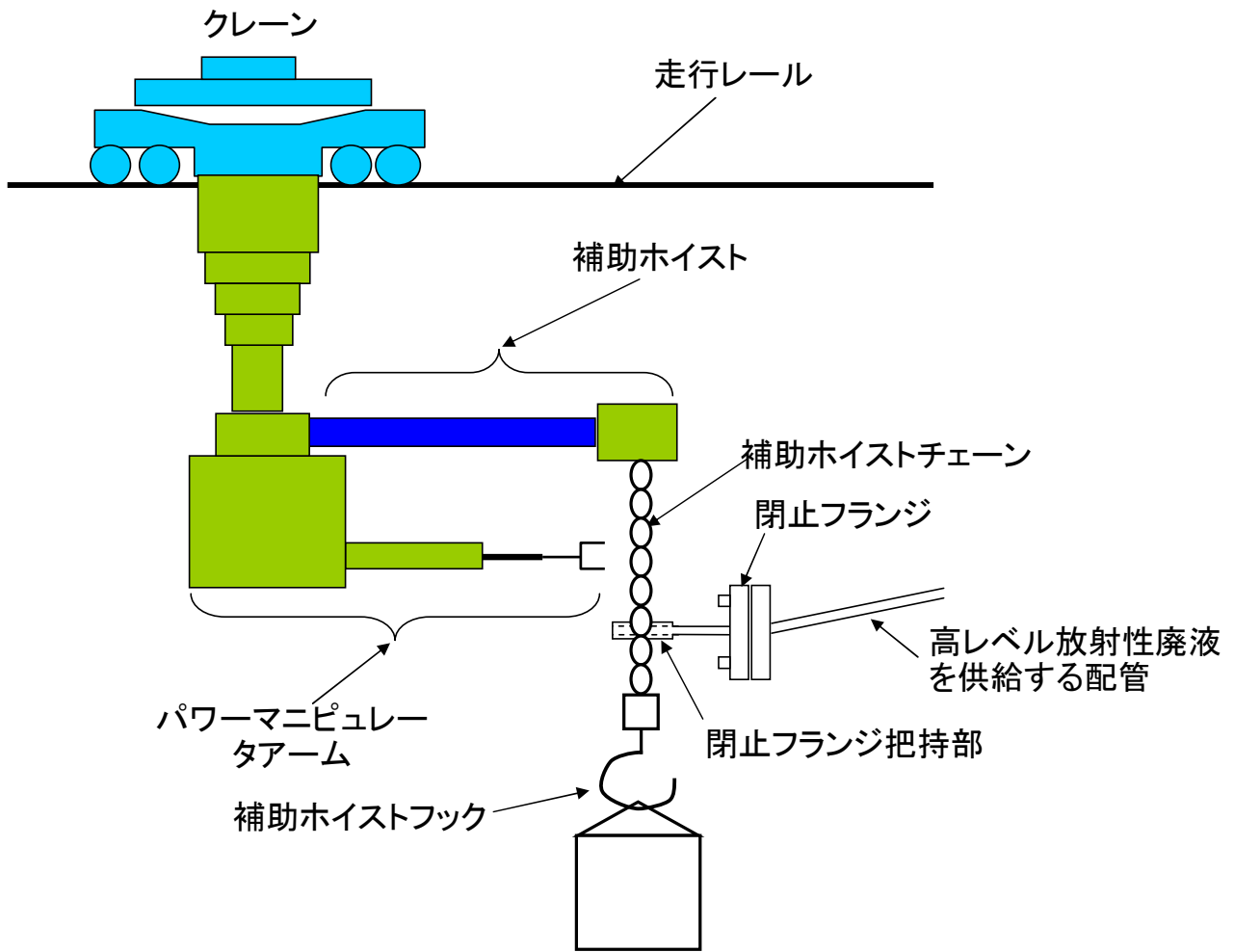
固化セル内の漏えいについての概要図
