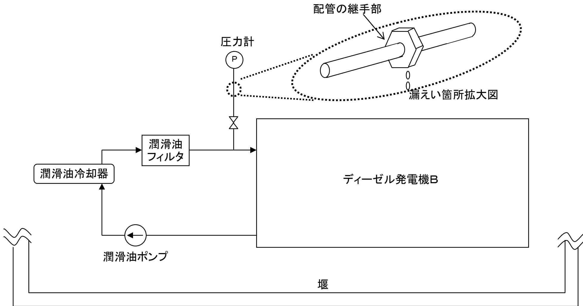
第1非常用ディーゼル発電機B室における潤滑油の漏えい概要図
