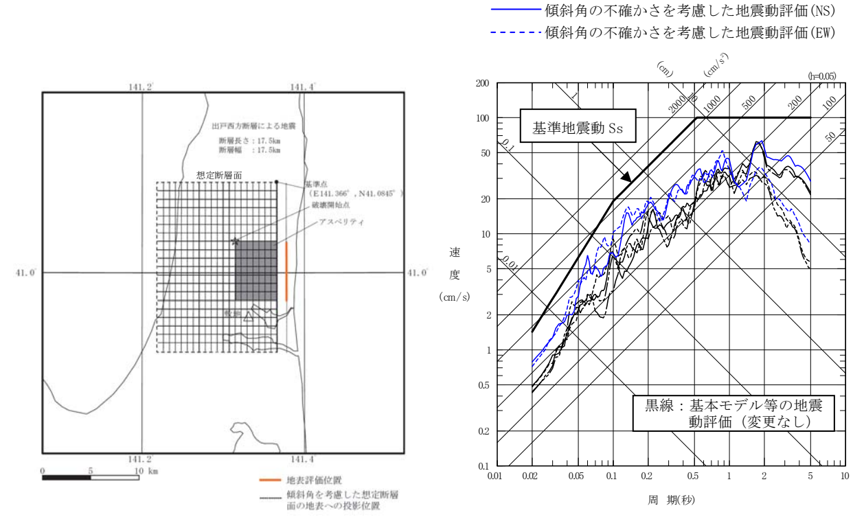
(a) 出戸西方断層による地震の断層モデル (傾斜角の不確かさを考慮した断層モデル)
