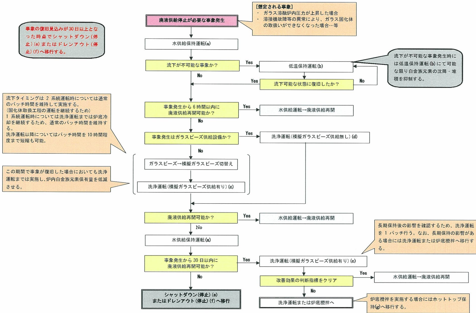
図一27 廃液供給停止が必要な事象発生時の対応（保持運転）フロー
