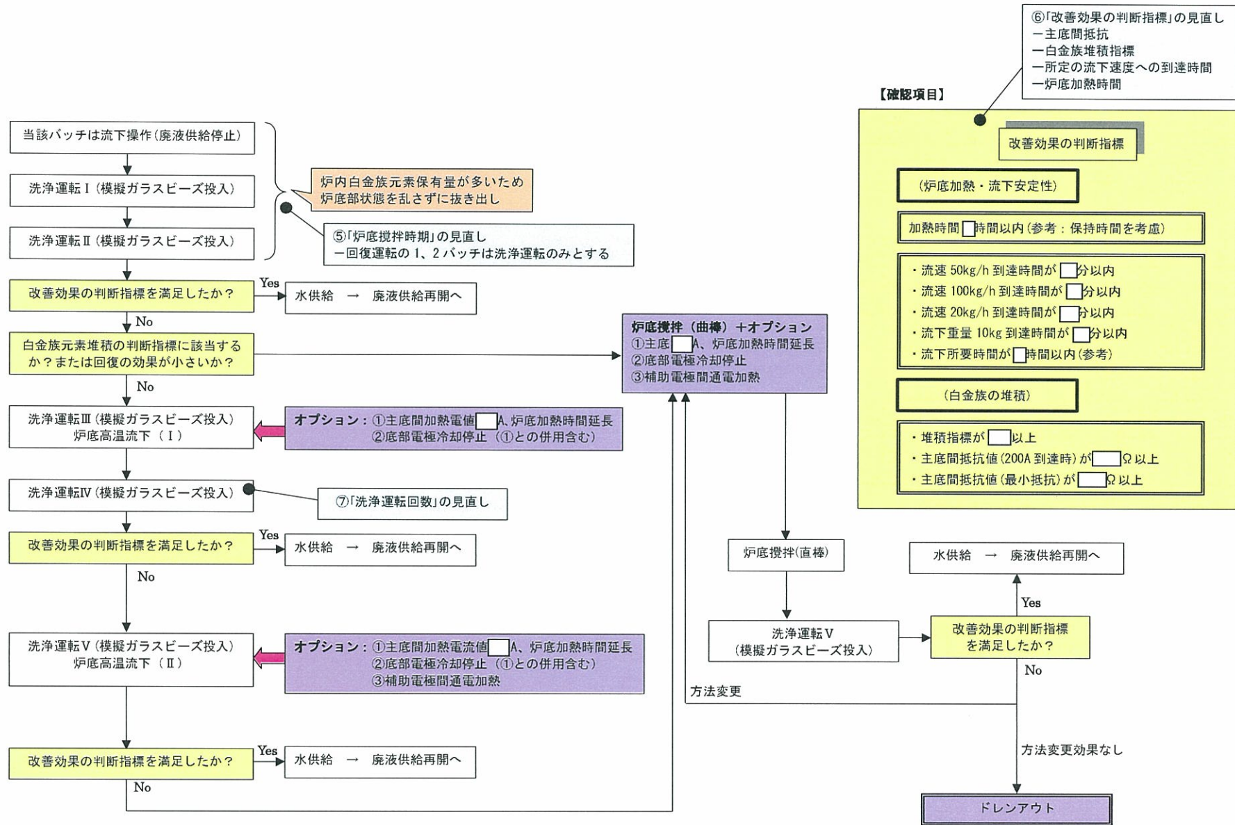
図—26 回復運転フロー
