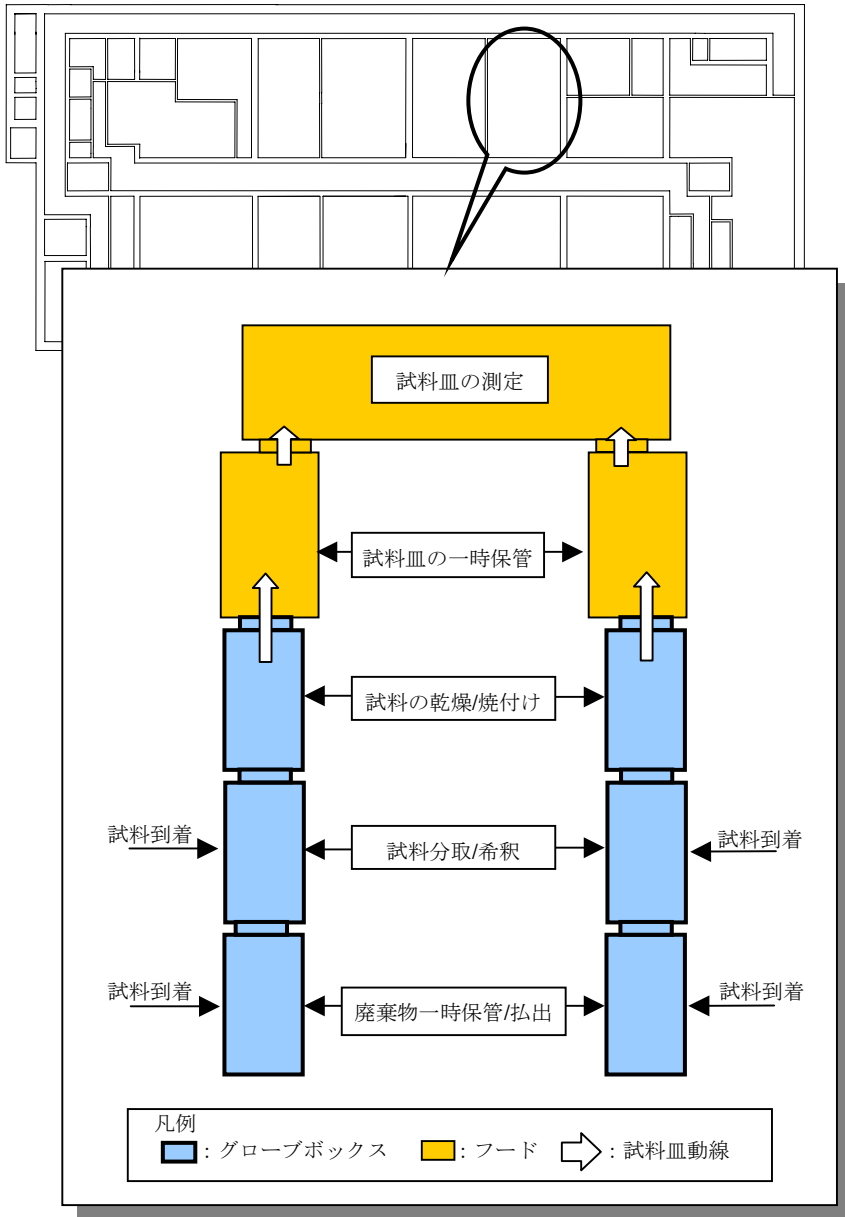
配置図
