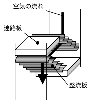
整流板：迷路板の間に設置し、冷却空気の流れの方向を整え、圧力損失を低減させる目的で設置する曲面の板。
