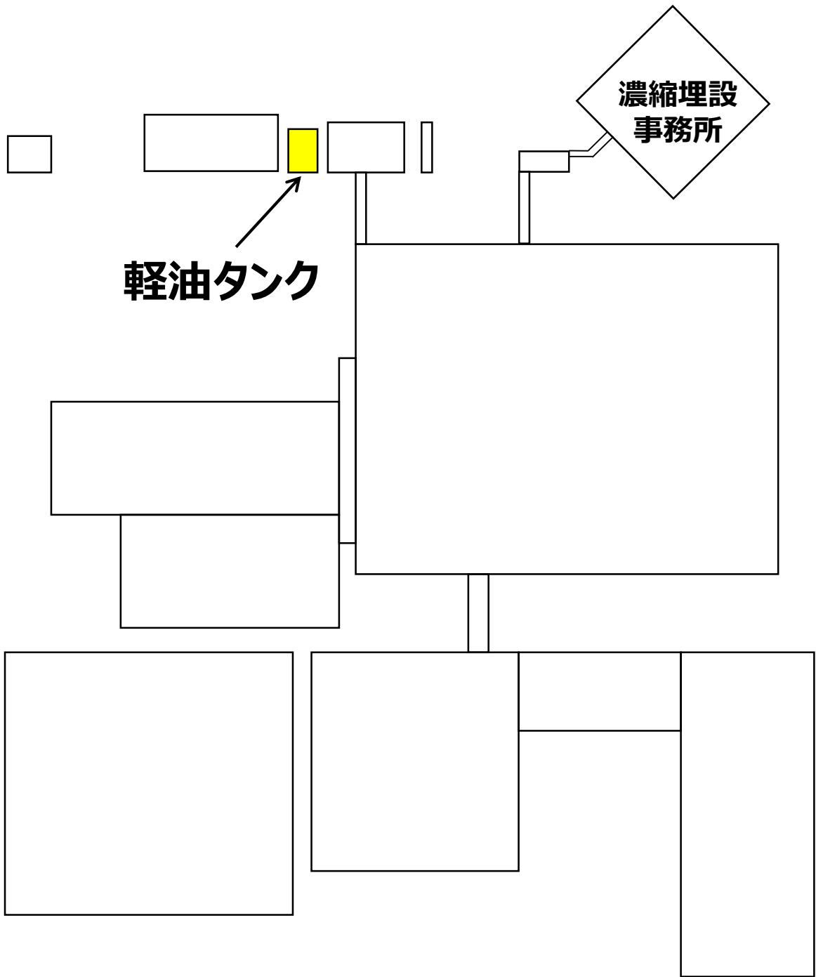
濃縮・埋設事業所 構内配置図
