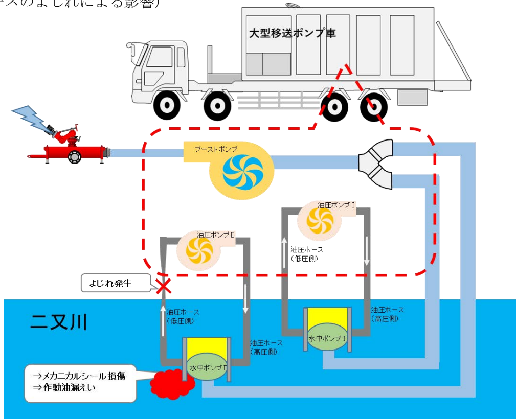
図2 (油圧ホースのよじれによる影響)
