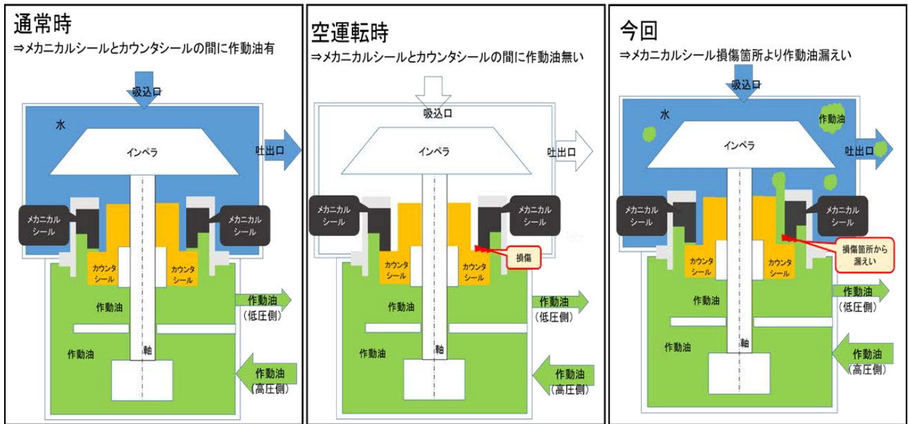
図1 (水中ポンプの空運転によるメカニカルシール損傷箇所からの漏えい)
