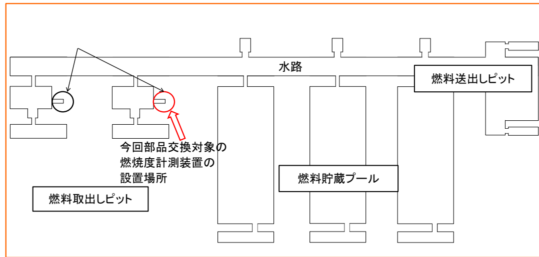
燃焼度計測装置の設置場所
