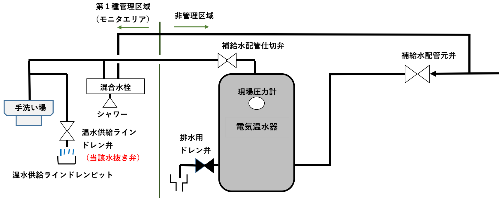
電気温水器系統 概略図
