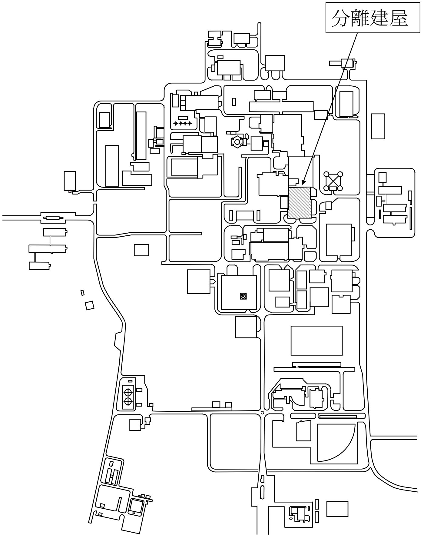
再処理事業所 構内配置図
