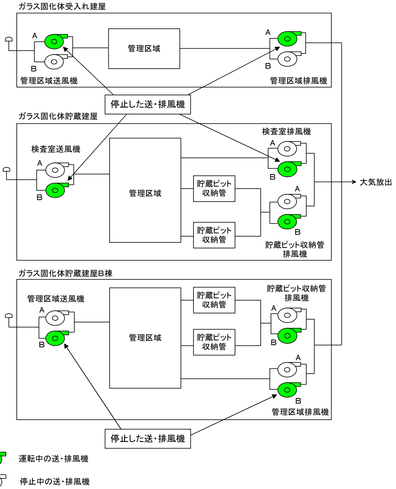
廃棄物管理施設の換気設備概要図
