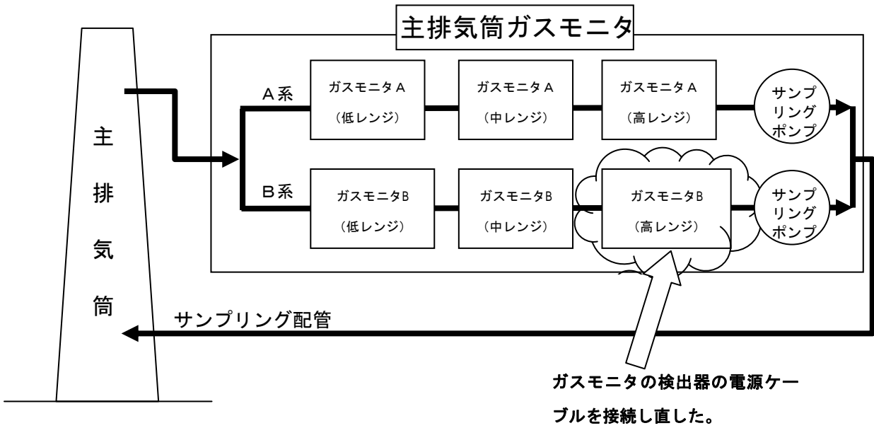
主排気筒ガスモニタ概要図
