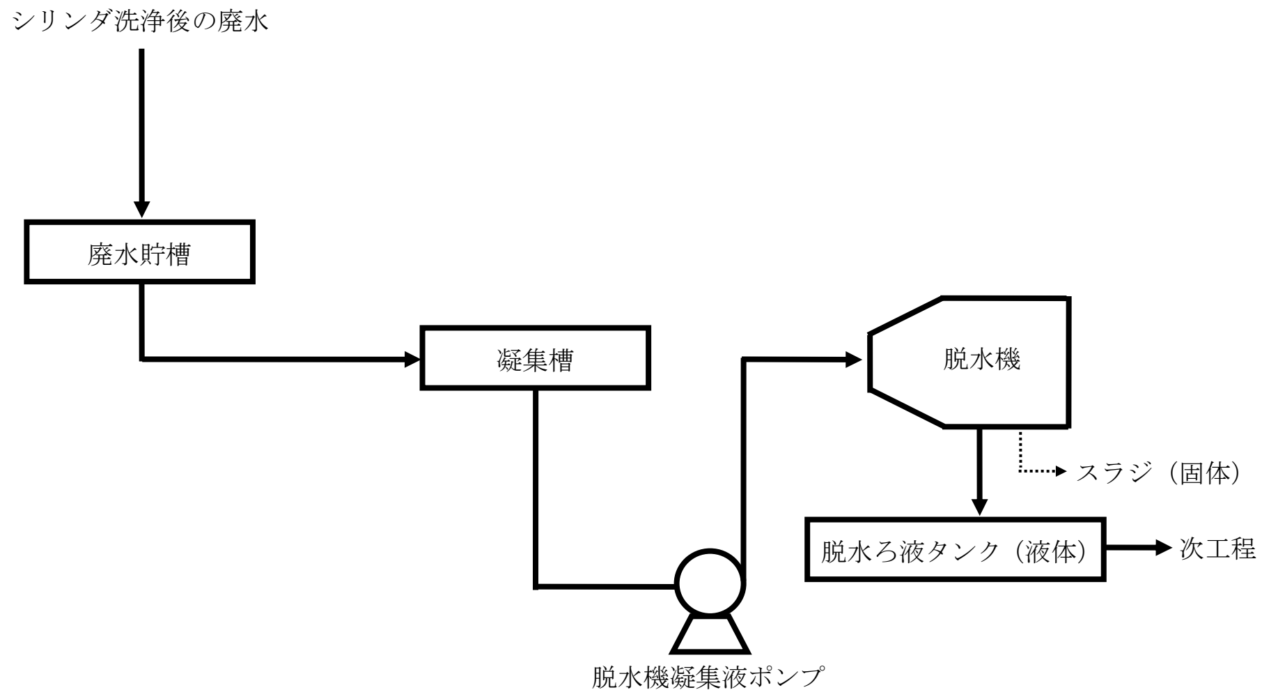
管理廃水処理設備 概略系統図
