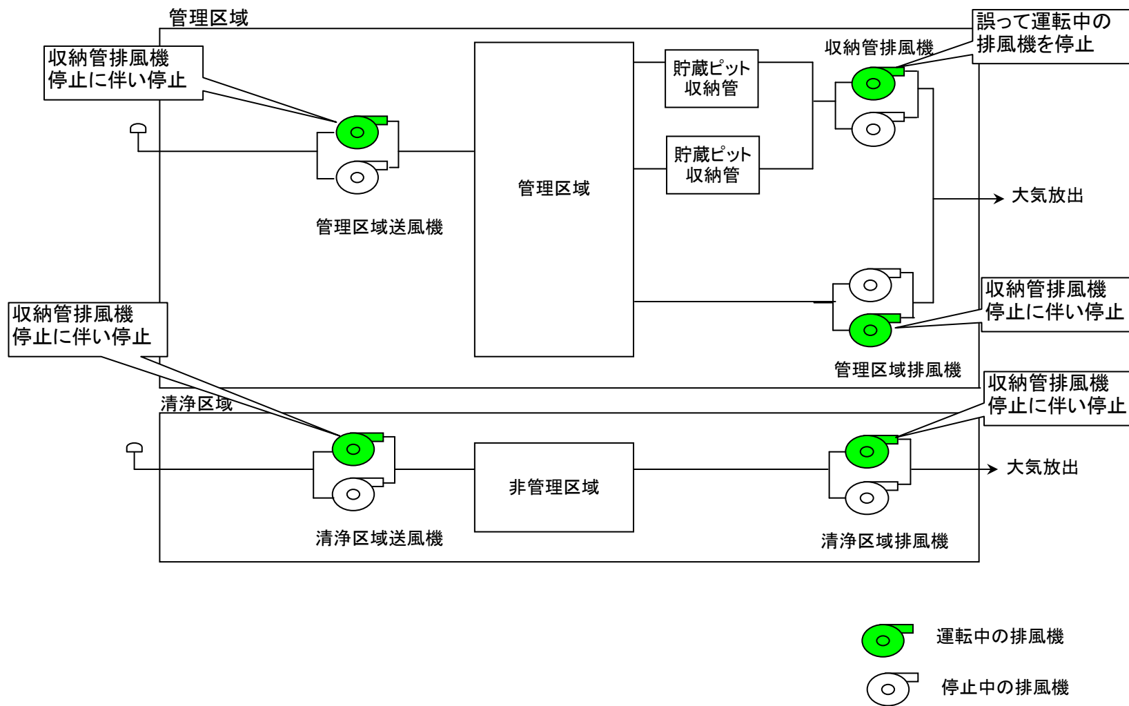
ガラス固化体貯蔵建屋B棟の換気設備概要図
