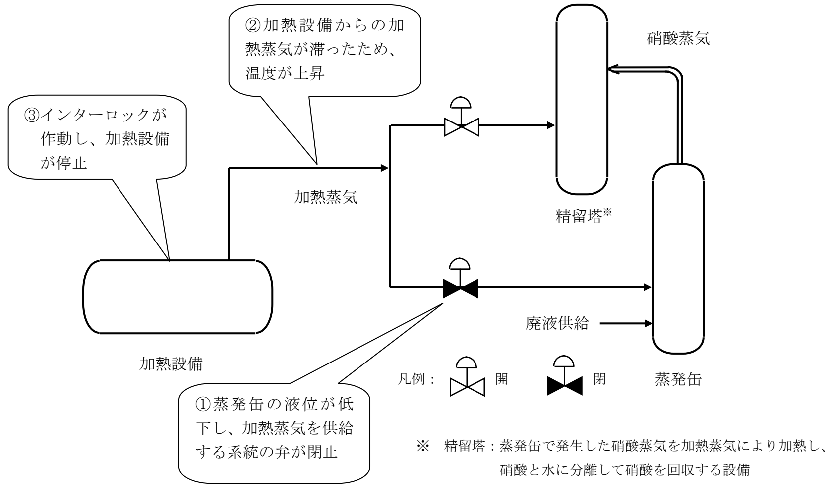
第2酸回収系設備概要図
