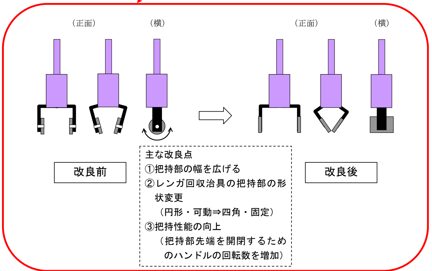
レンガ回収治具の改良概要図
