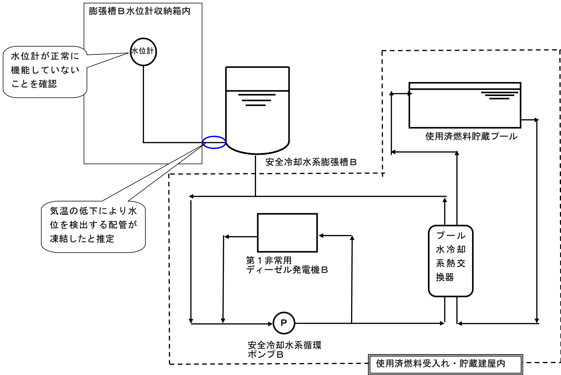
安全冷却水系系統概要図
