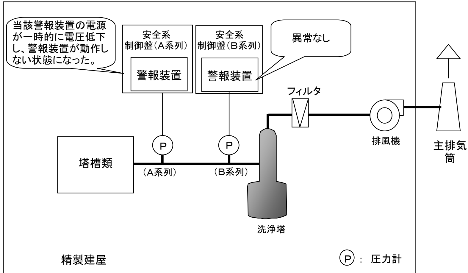
塔槽類廃ガス処理設備系統概要図
