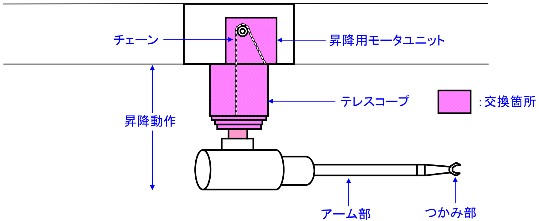
固化セルパワーマニピュレータ 概要図
