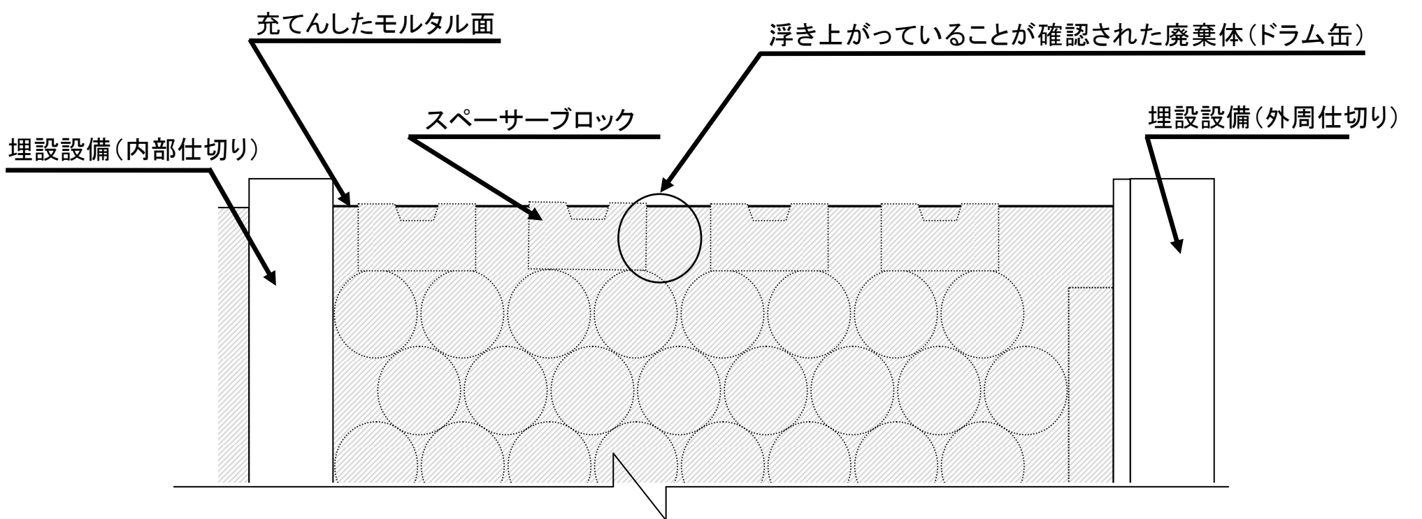
概要図(推定断面図)
