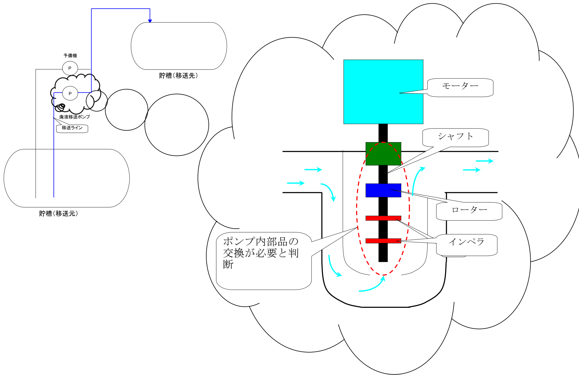
廃液移送ポンプ概要図
