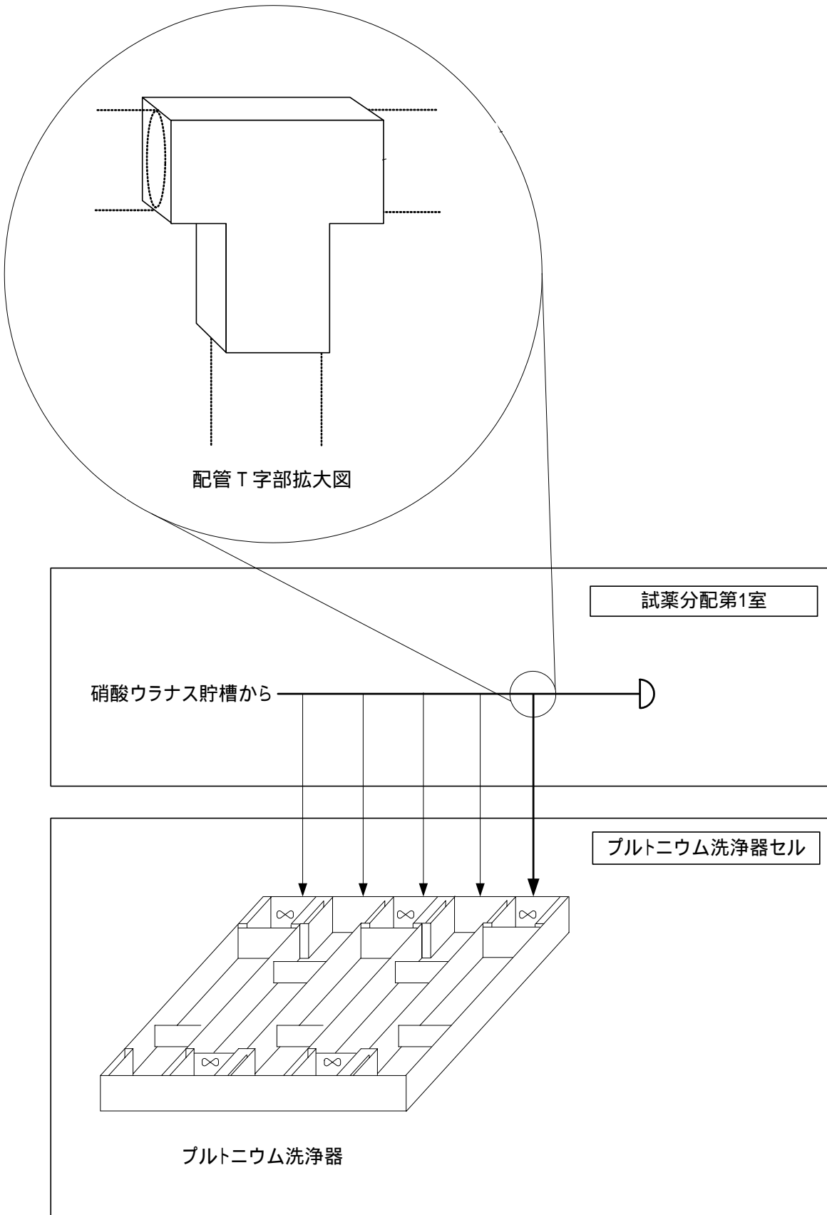
漏えい箇所概要図
